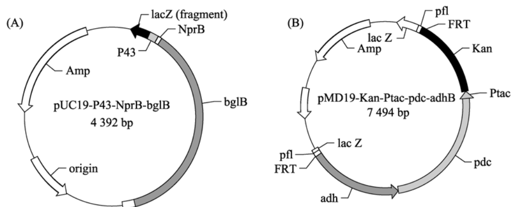
图 2 T- kan-P tac -pdC-adhB 与 pUC19- P_{43} - NprB-bglB 的质粒图谱
